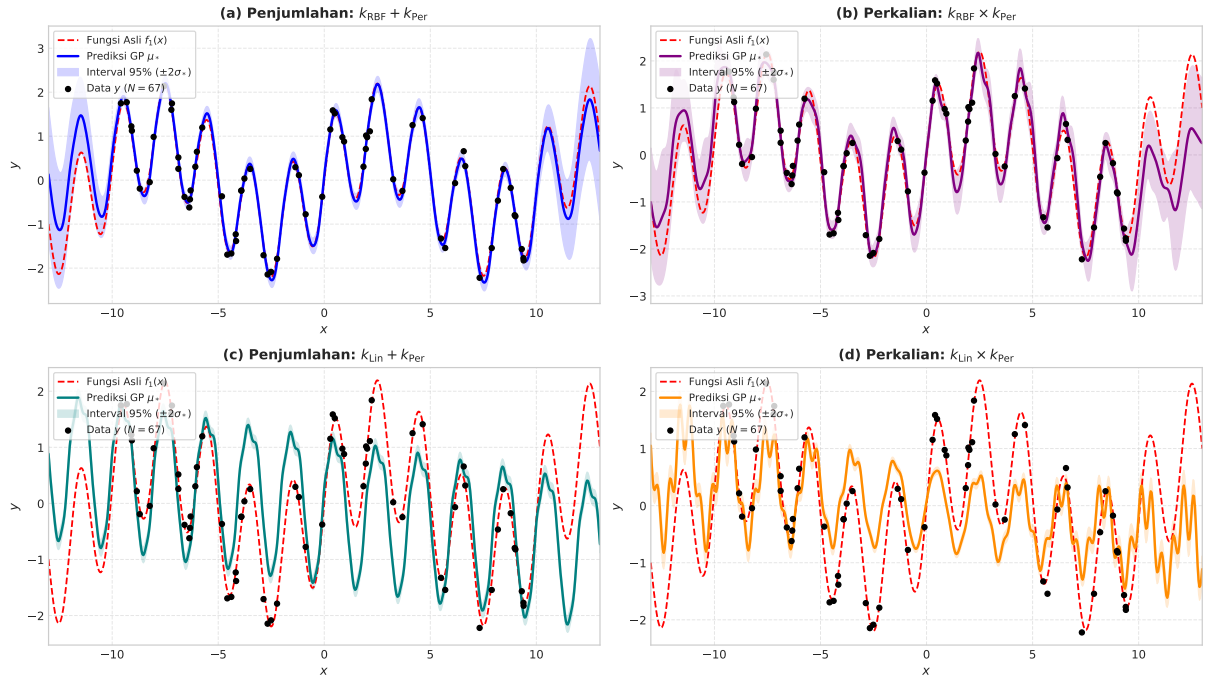
Gambar 2: Hasil fitting Gaussian Process Regression pada fungsi asli f_1(x) (36): (a) k_{\text{RBF}} + k_{\text{Per}} ; (b) k_{\text{RBF}} \times k_{\text{Per}} ; (c) k_{\text{Lin}} + k_{\text{Per}} ; (d) k_{\text{Lin}} \times k_{\text{Per}} .
