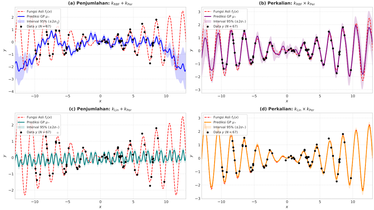
Gambar 3: Hasil fitting Gaussian Process Regression pada fungsi asli f_2(x) (37): (a) k_{\text{RBF}} + k_{\text{Per}} ; (b) k_{\text{RBF}} \times k_{\text{Per}} ; (c) k_{\text{Lin}} + k_{\text{Per}} ; (d) k_{\text{Lin}} \times k_{\text{Per}} .
